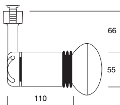
PAR 20
